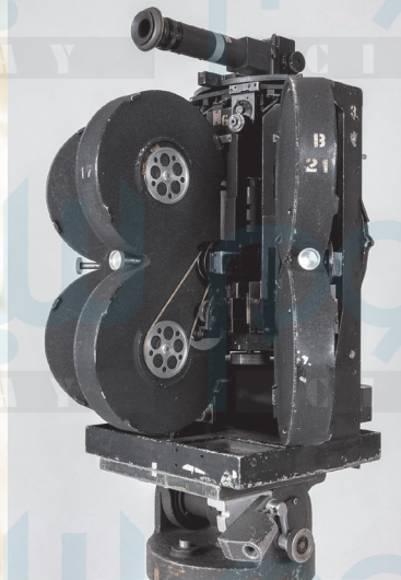
كاميرا ثلاثية البكرات الخاصة في تصوير (السيناراما).
