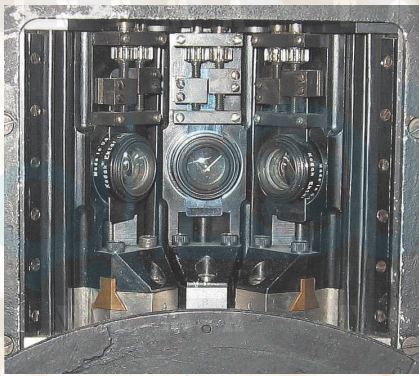
عدسات الكاميرا ثلاثية البكرات الخاصة في تصوير (السيناراما).
