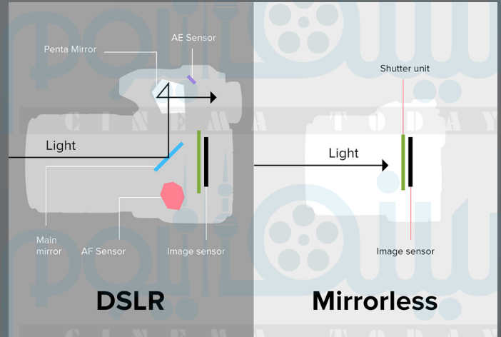
صورة توضيحية للفرق بين نظام كاميرا (DSLR) و نظام كاميرا (Mirrorless).
